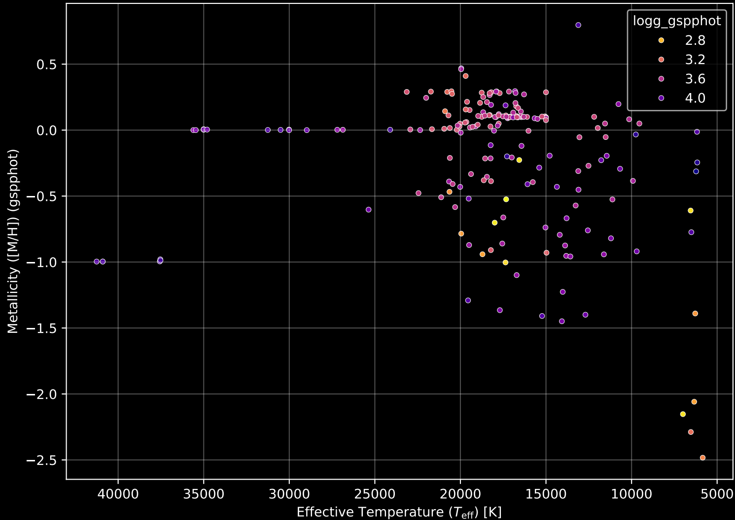
APOGEE DR17 Field: [135-03] Stellar Population Parameters (n= 195)
